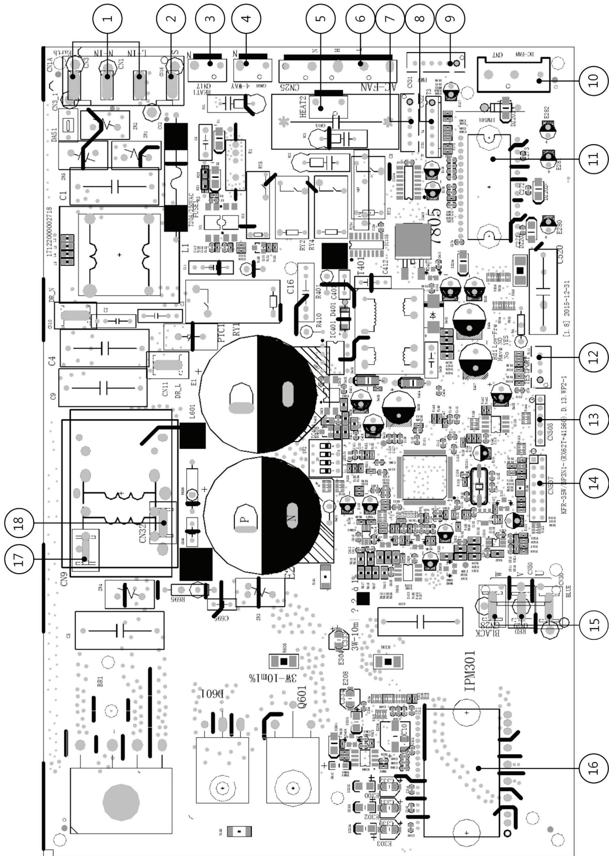
Схема печатной платы наружного блока 17122000038329
